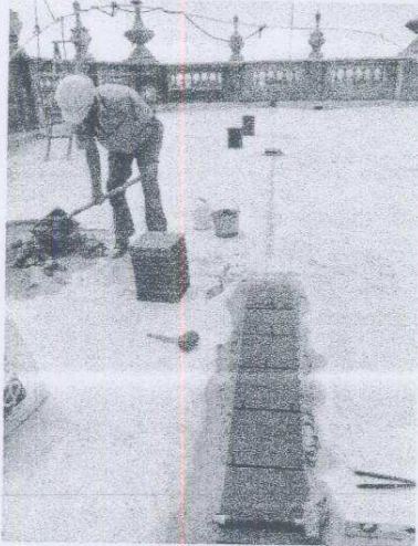
Colocación de Cinteado para guía ("maestras")
